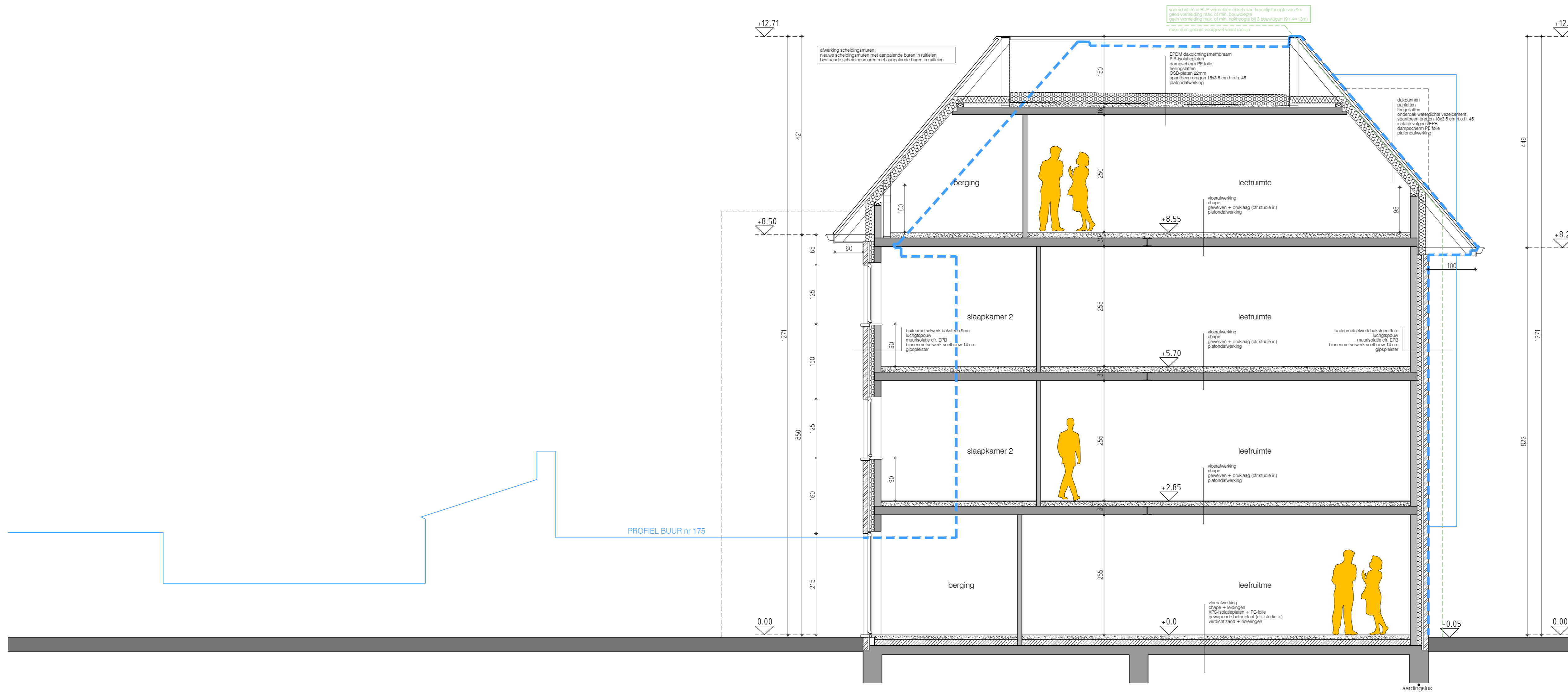
doorsnede 2-2
